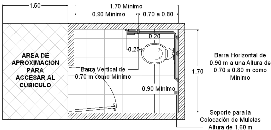
PLANTA
