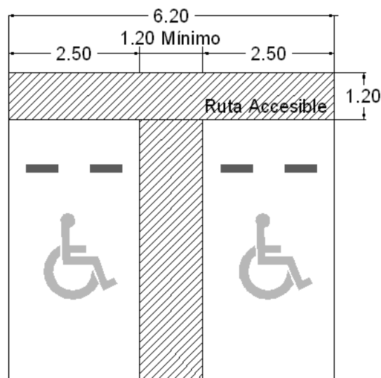
PLANTA ARQUITECTONICA
