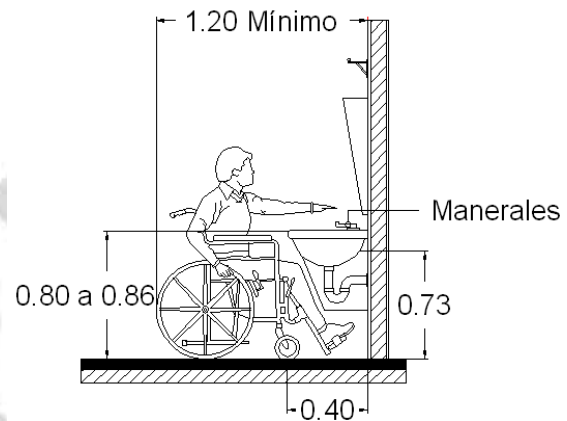
ALZADO LATERAL
