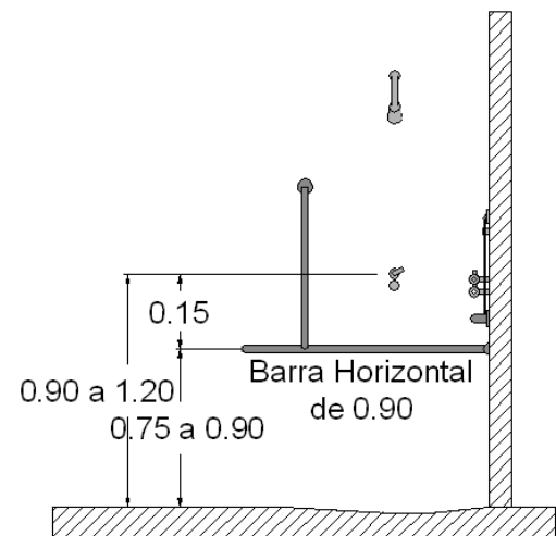
ALZADO LATERAL
