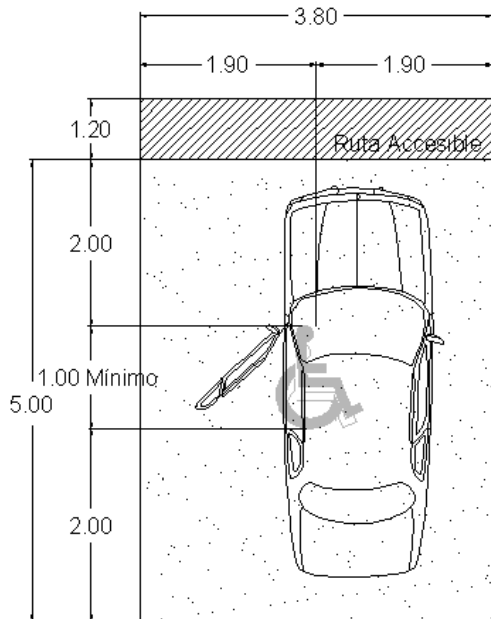
PLANTA ARQUITECTONICA
