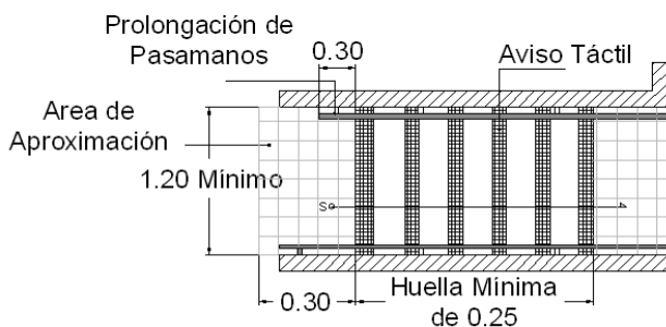
PLANTA ARQUITECTONICA
