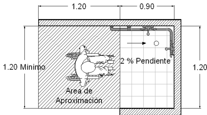
PLANTA
