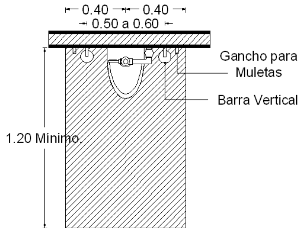
PLANTA ARQUITECTONICA
