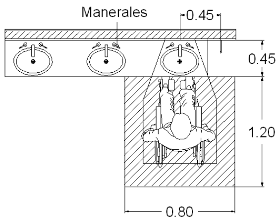
PLANTA ARQUITECTONICA
