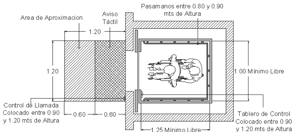
PLANTA ARQUITECTONICA
