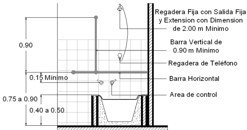
ALZADO LATERAL
