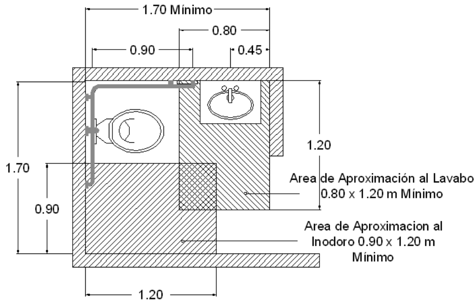
PLANTA ARQUITECTONICA
